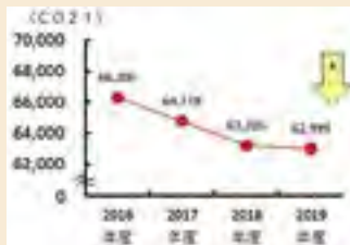
CO 2 排出量
